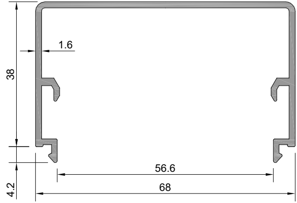
Profil No: ÇT68-303 Ağırlık : 750 gr/m
